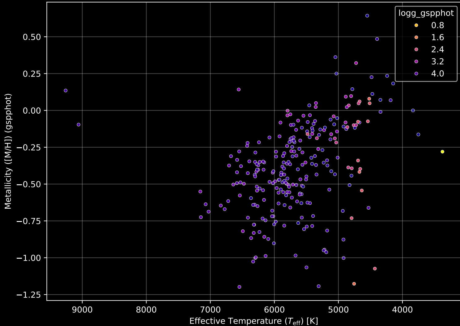
GALAH DR4 Field: [1107] Stellar Population Parameters (n= 257)
