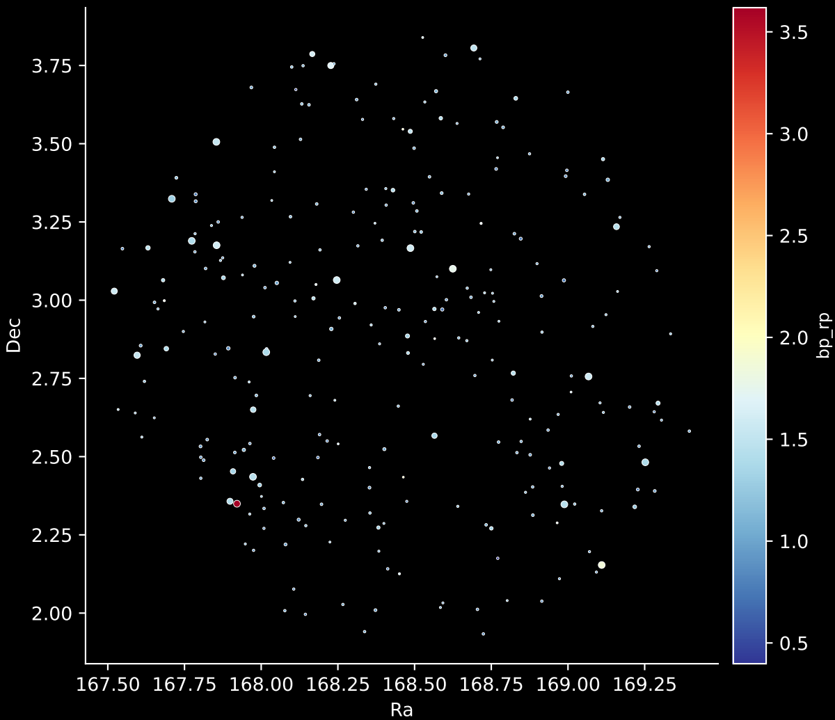
GALAH DR4 Field: [1107] Stars: 257
