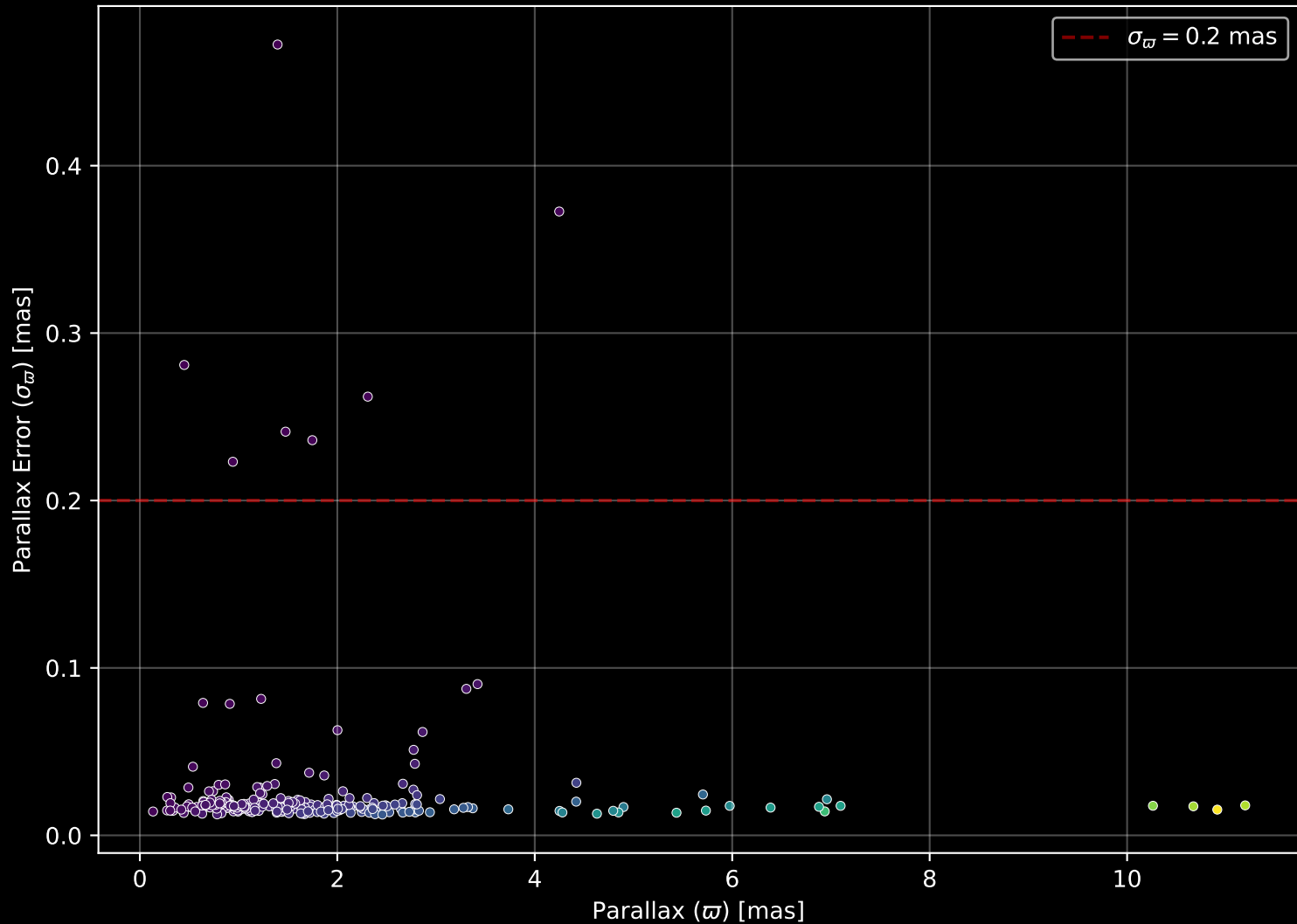
GALAH DR4 Field: [1107] Parallax Quality (n= 257)
