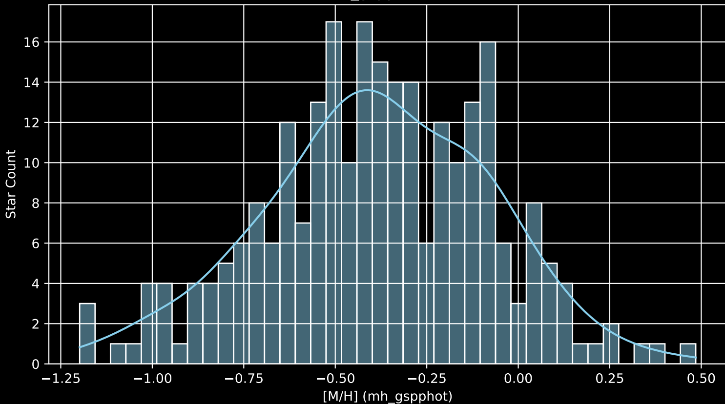
GALAH DR4 Field: [1107] [M/H] (mh_gspphot) (n= 256)
